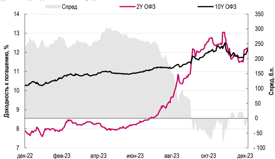
Динамика доходностей ОФЗ и спред 10-2
